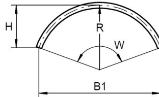
Stichbogen
